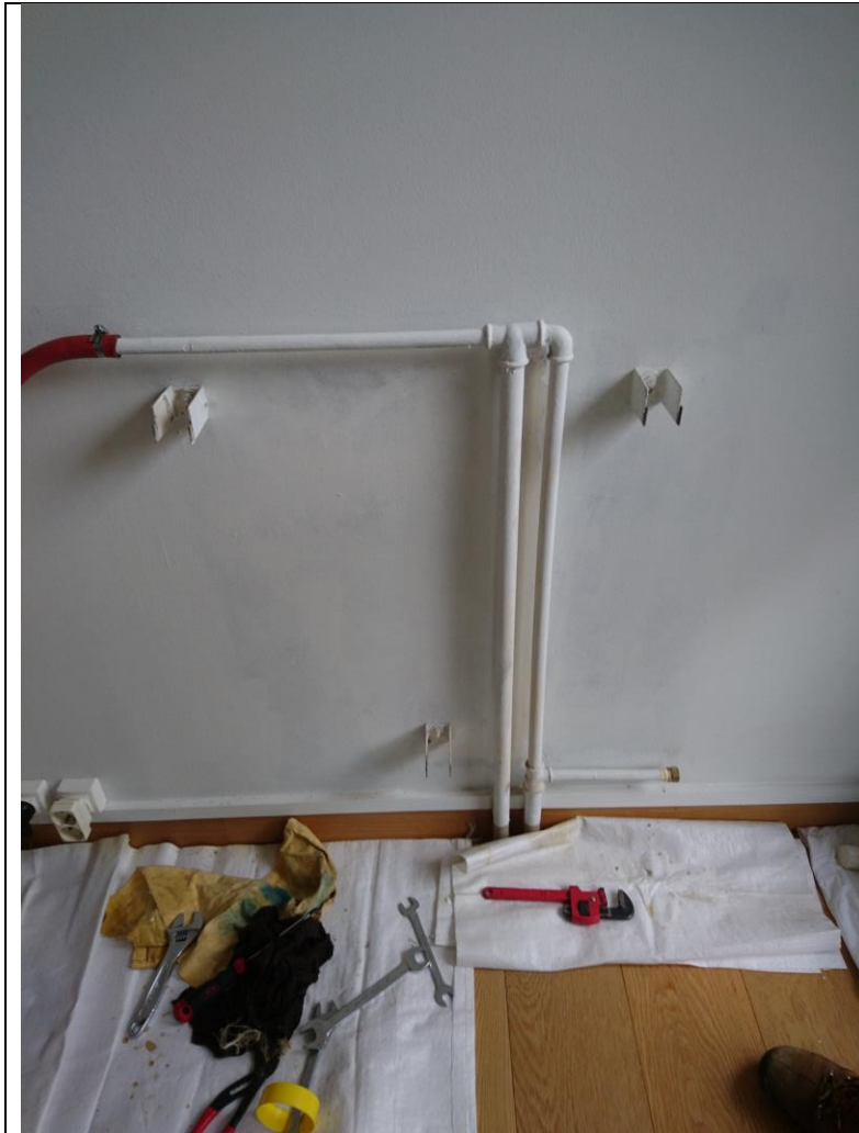
Alimentation standard de radiateur
